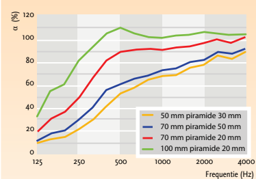
Geluidsabsorptiewaarden
